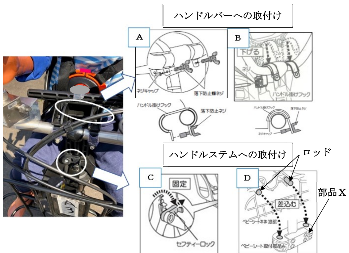
図 65 ハンドル部への前座席の取付方法 (左：座席 A、右：座席 B)
