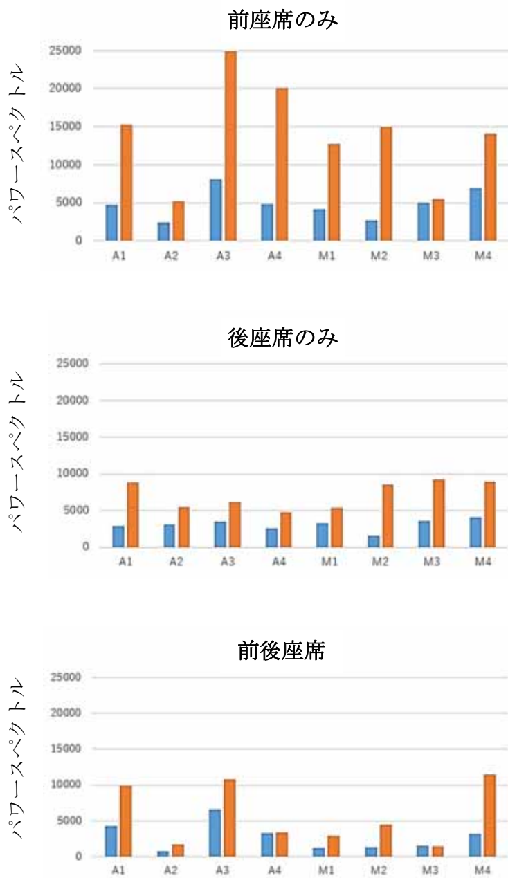
図 50 ダミー人形乗せ位置別の評価結果（周波数解析） ※棒グラフは、左：フラット（エリア0）、右：段差5cm（エリア2）
