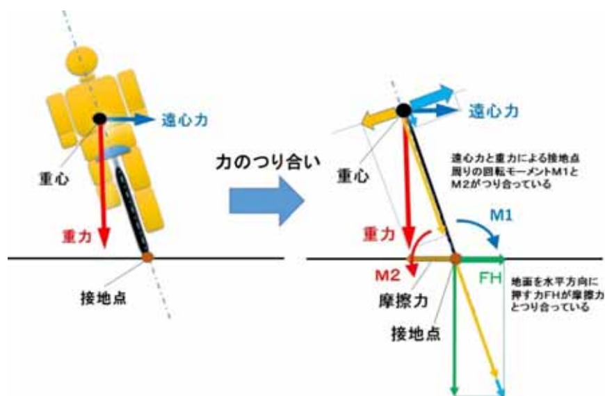
図 37 走行中の自転車のバランス
