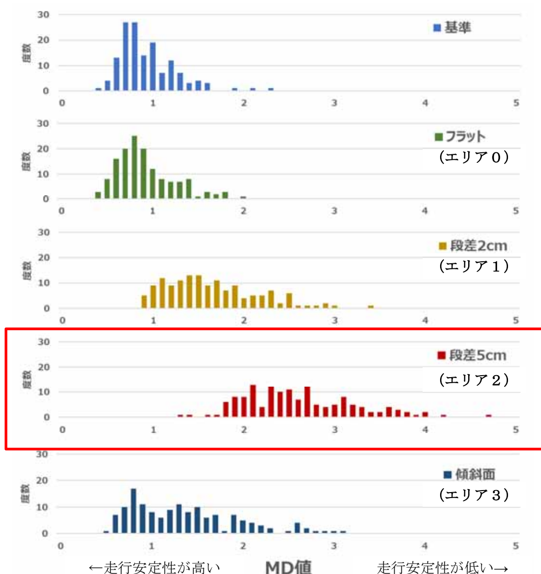
図 44 エリア別の評価結果
