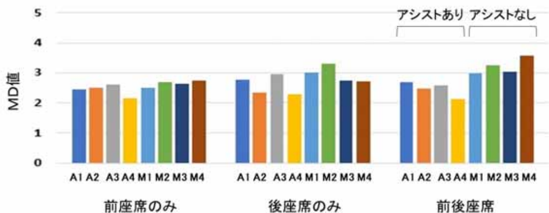
図 47 ダミー人形乗せ位置別の評価結果（MT 法：段差 5 cm）
