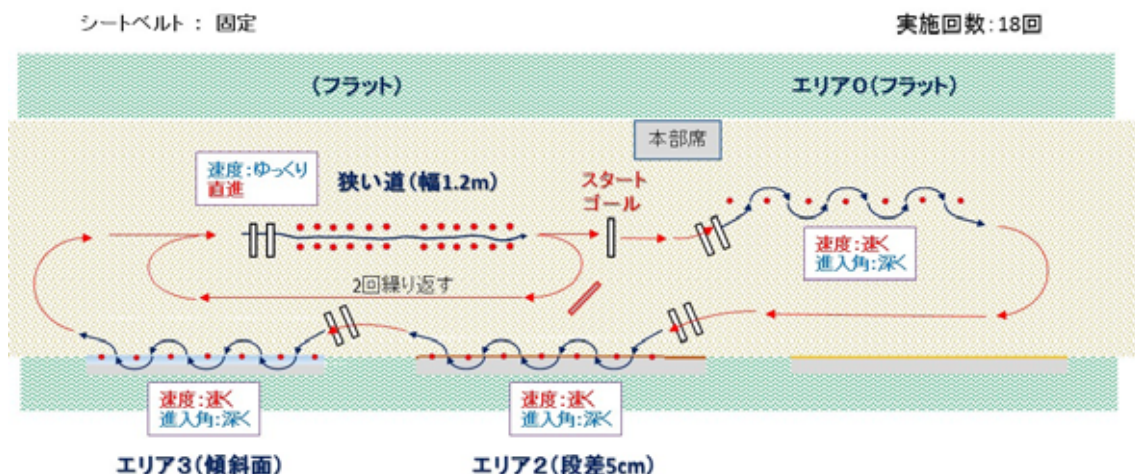
図 62 走行方法（実験C）
