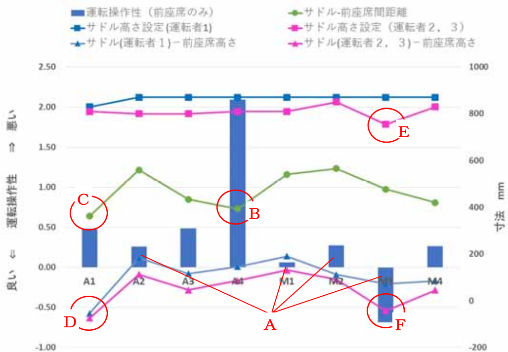
図 55 運転操作性と前座席及びサドルの位置関係（ダミー人形前座席のみ） （寸法関係は右側の第 2 軸で示す。）
