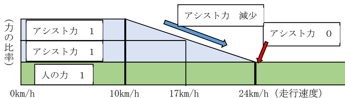
図5 アシスト比率
