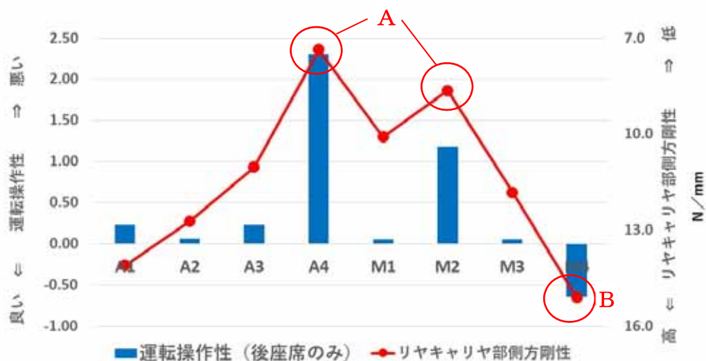
図 57 運転操作性とリヤキャリヤ部剛性との関係 (ダミー人形後座席のみ)
