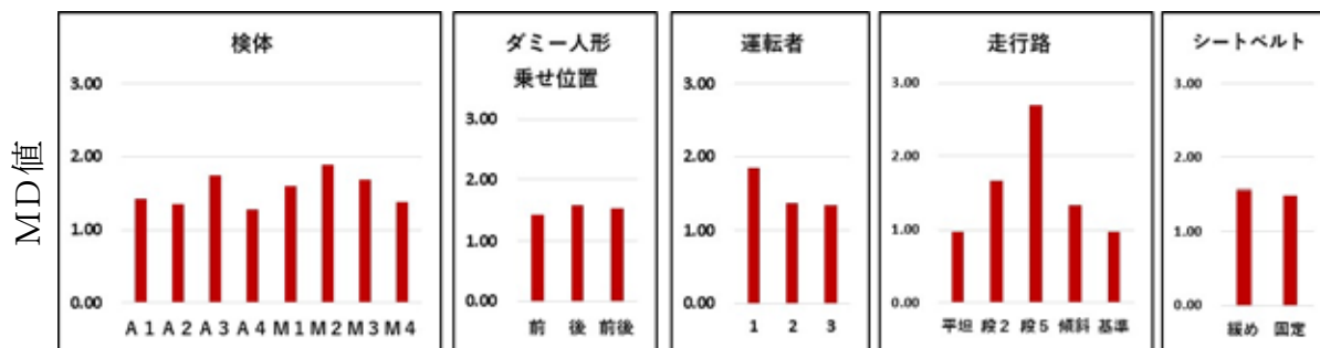
図45 要因別の評価結果（全体）
