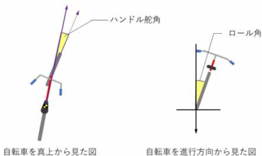
図 38 ハンドル舵角及びロール角
