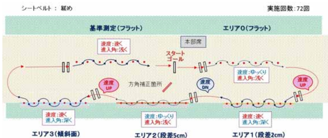
図 43 走行方法（実験 A II：組合せ水準 N 5～N 8）
