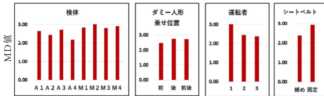
図 46 要因別の評価結果（段差 5 cm）
