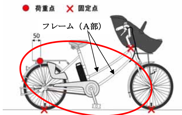
図 56 リヤキャリヤ部（赤枠）と剛性測定方法
