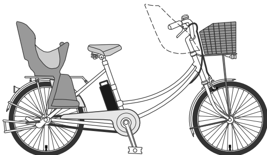
図3 後ろ乗せタイプの幼児乗せ自転車
