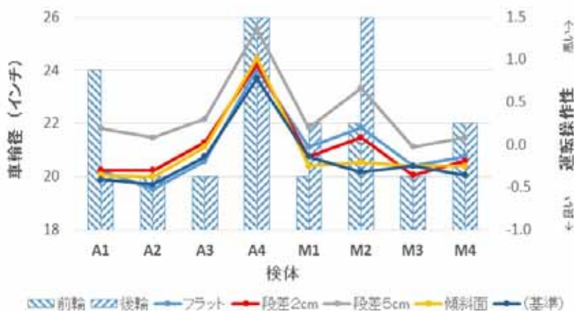
図 53 各検体の車輪径と運転操作性の評価結果 (実験 A)
