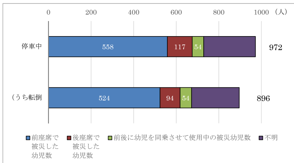
図 12 停車中の事故の被災幼児座席内訳
