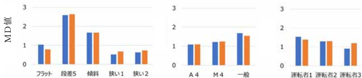
図 63 要因別の荷物の載せ方の違いによる評価結果
