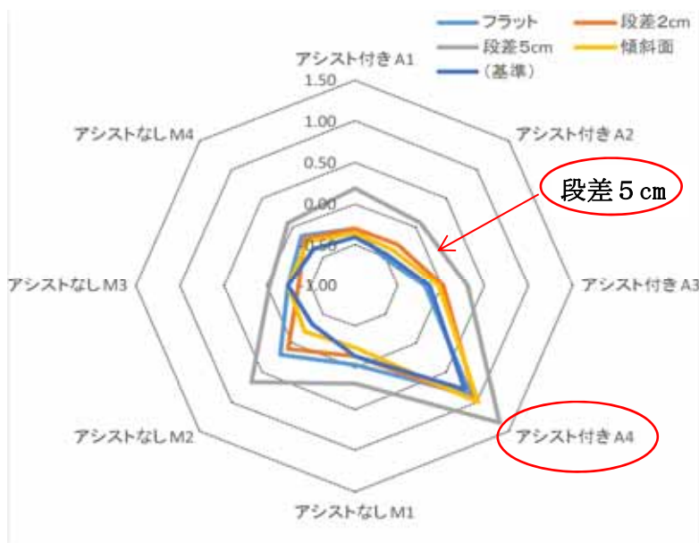
図 52 検体別運転操作性の評価結果 (実験 A)
