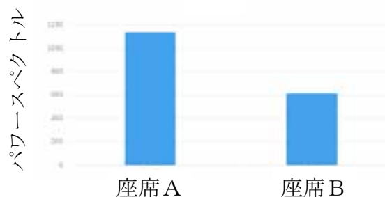
図 69 ハンドル舵角の周波数解析結果（フラット）
