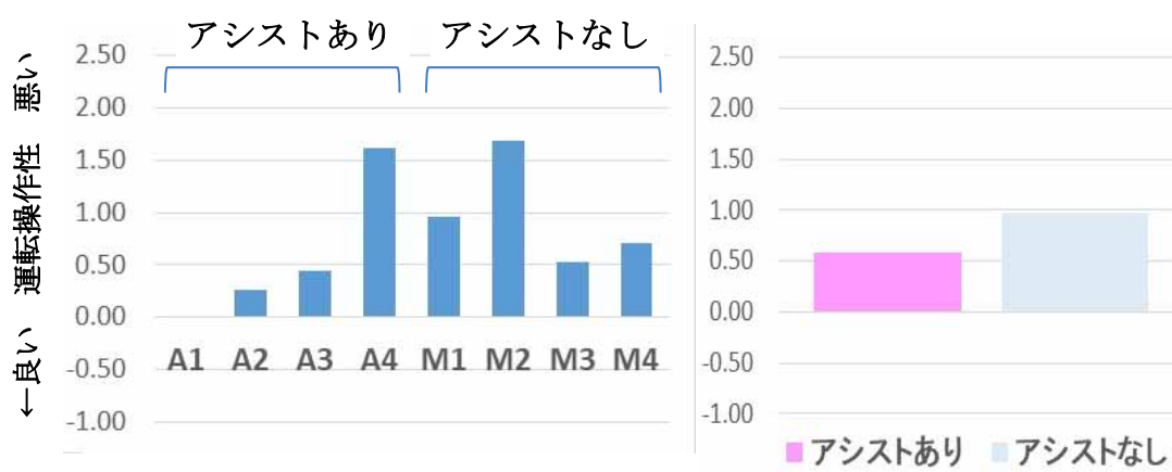
図 59 運転操作性（ダミー人形前後座席）
