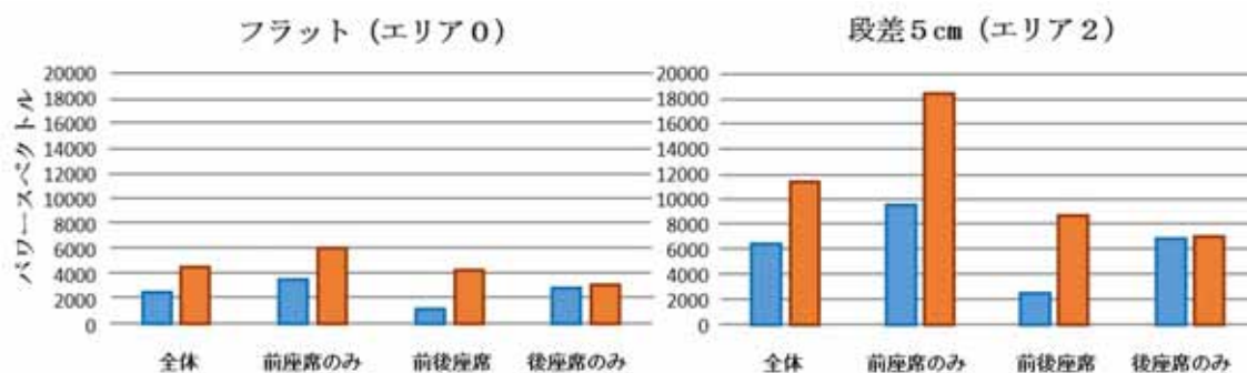
図 51 ダミー人形乗せ位置別の自転車タイプの評価結果 ※棒グラフは、左：前乗せタイプ、右： 後ろ乗せタイプ
