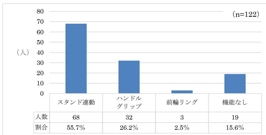
図29 ハンドルロックの種類
