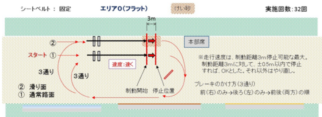
図 64 走行方法（実験D）
