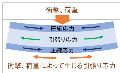
図1 強化ガラスの断面イメージ
